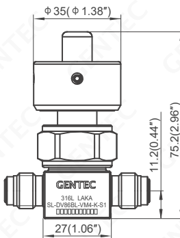
手动 (300 psi) 手柄式, 带开关显示
