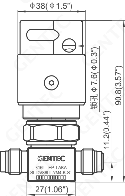
手动 (300 psi) 条形式, 带锁, 带开关显示
