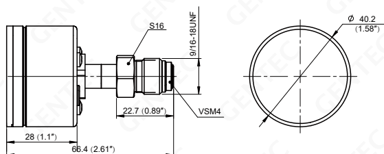
GUR15SL-*-VSM4
